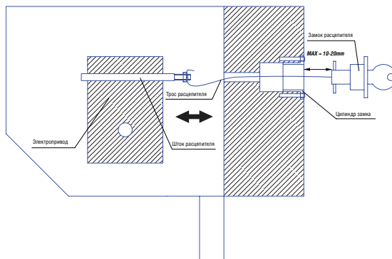
Рис.6б. Вывод управления через стену
