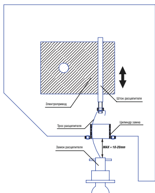
Рис.6а. Вывод управления из короба
